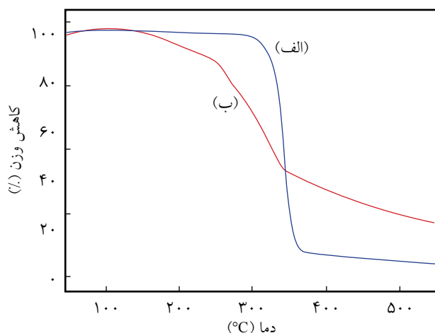
شکل ۴- دمانگاشت DSC: (الف) سلولوز و (ب) ترپلیمر آکریلونیتریل-۴- کلرومتیل استیرین-سلولوز.
