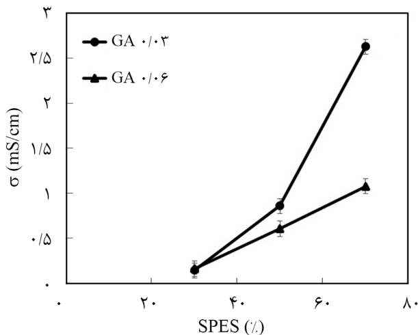
شکل ۴- هدایت پروتون ترکیب‌های مختلف غشای تبادل پروتون.
