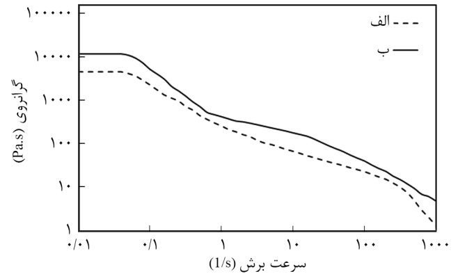
شکل ۱۰- نمودار گرانشی برحسب سرعت برش در آزمون برشی پایا: (الف) پلی‌وینیل استات خالص و (ب) پلی‌وینیل استات دارای ۱/۵٪ نانوذرات سیلیکای کلئیدی.
