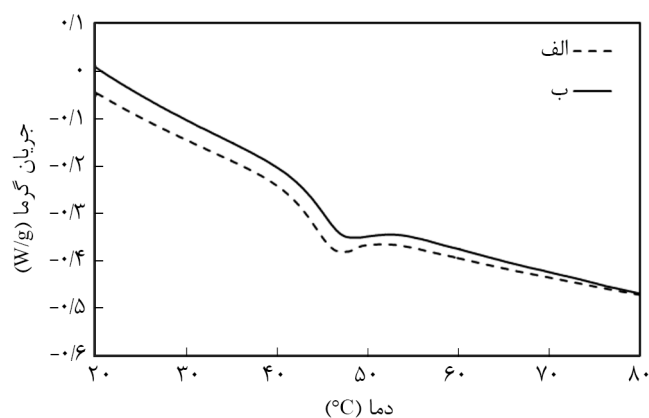
شکل ۵- دمانگاشت DSC: (الف) پلی وینیل استات خالص و (ب) پلی وینیل استات دارای ۱/۵٪ نانوذرات سیلیکای کلونیدی.
