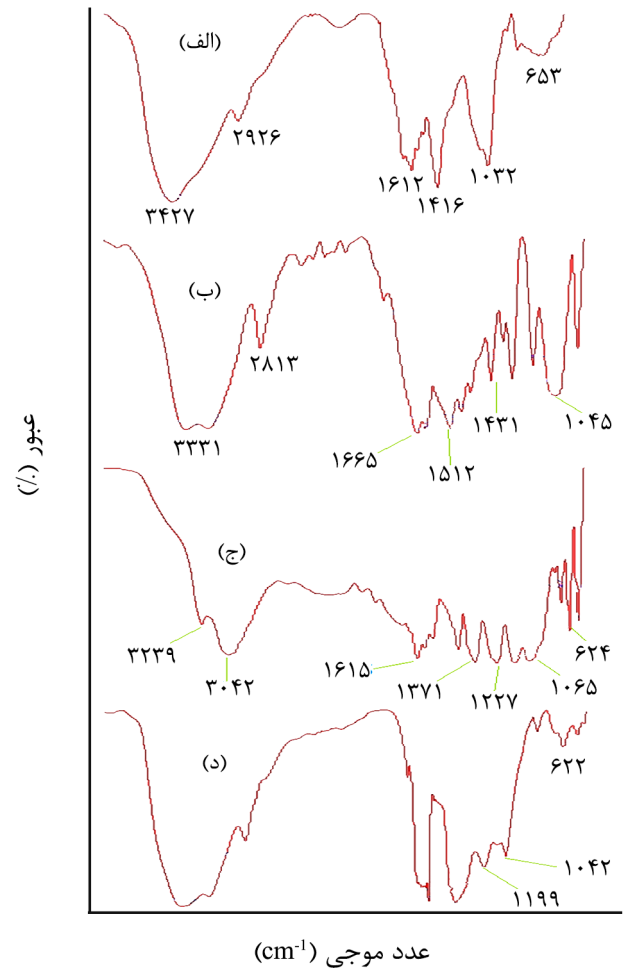
شکل ۱- طیف FTIR: (الف) سدیم آلزینات، (ب) مونومر AA، (ج) مونومر AMPS و (د) هیدروژل نانوکامپوزیتی.
