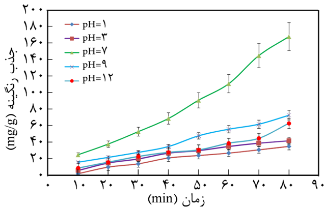
شکل ۷- اثر pH اولیه محلول رنگینه بر جذب رنگینه آبی متیلن به وسیله هیدروژل نانوکامپوزیتی (شرایط جذب رنگینه AgNO_3=80 mg, AMPS=5 g, AA=3 mL, V=10 mL, W=3 g, T=45^\circ C , t=60 min, C_0=100 mg/L).
