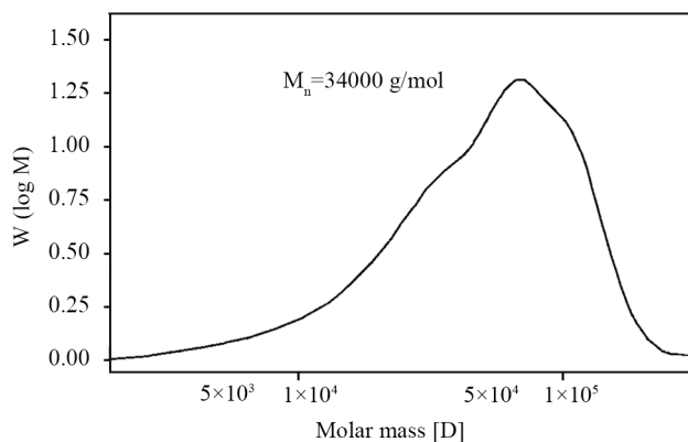
شکل ۳- توزیع وزن مولکولی پلی(هگزیل متاکریلات) در ۷۰°C، ۰/۲۵٪ وزنی آغازگر و ۹۰٪ وزنی حلال.
