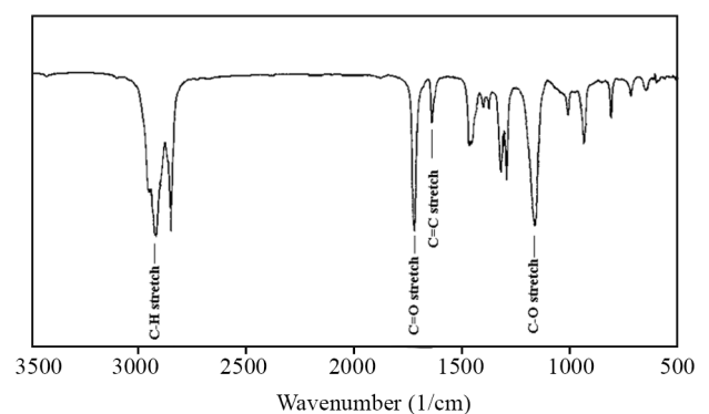
شکل ۱- طیف FTIR دسیل متاکریلات سنتزی.
