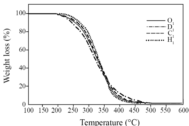
شکل ۴- گرمانگاشت TGA پلی (آلکیل متاکریلات)های سنتزی: پلی (اکتیل متاکریلات)، ( O_1 ) پلی (دودسیل متاکریلات)، ( H_1 ) پلی (هگزیل متاکریلات) و ( C_1 ) پلی (دودسیل متاکریلات).
