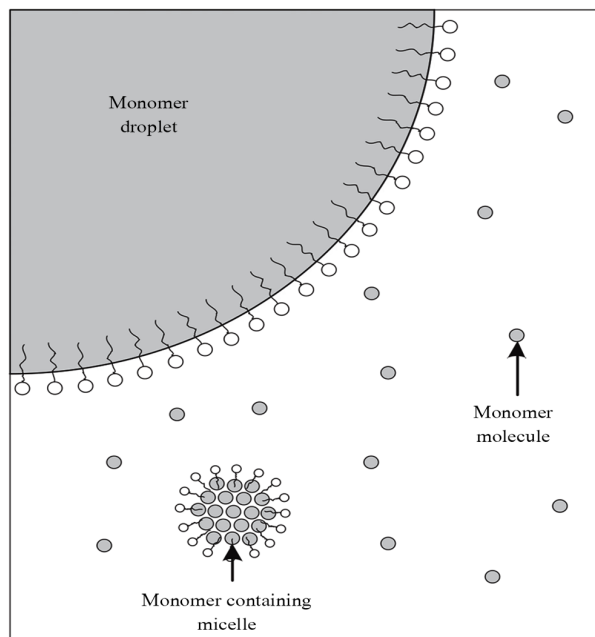
شکل ۱۴- طرحی از مراحل اولیه پلیمر شدن امولسیونی [۳۴].
