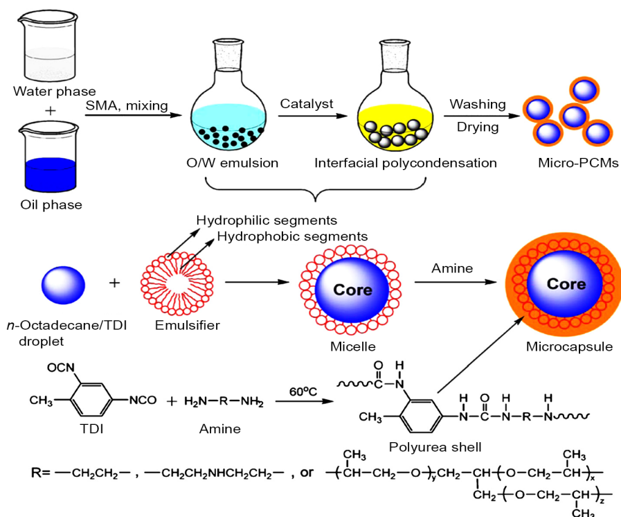
شکل ۱۰- طرحی از تشکیل n-اکتادکان میکروکپسول‌دار شده با پوسته‌های پلی‌اوره دارای قطعه‌های نرم مختلف از پلیمر شدن تراکمی بین‌سطحی [۳۹]. Fig. 10. Schematic formation of the microencapsulated n-octadecane with the polyurea shells containing different soft segments through interfacial polycondensation [39].
