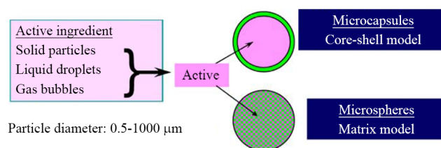
شکل ۵- ساختار مواد تغییر فاز میکروکپسول‌دار شده (MEPCMs) [۳۵].
