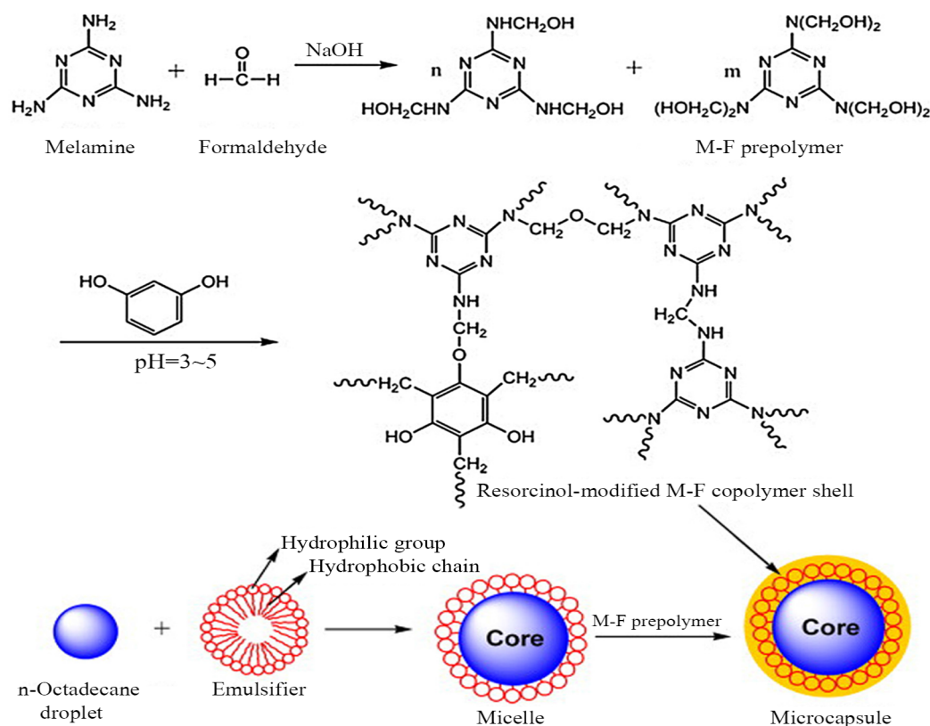
شکل ۱۱- طرحی از تشکیل PCMهای میکروکپسولی بر پایه هسته n-اکتادکان و پوسته پلی (ملامین-فرمالدهید) اصلاح شده به کمک رزورسینول با پلیمر شدن درجا [۵۵].
