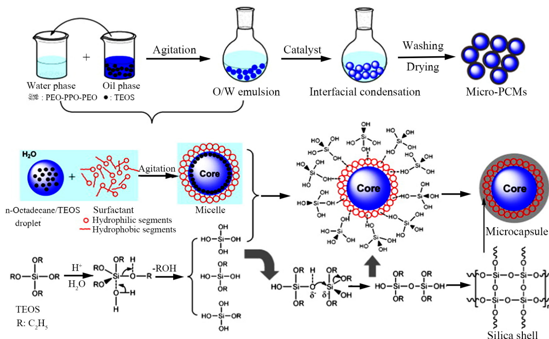
شکل ۹- طرحی از ساخت میکروکپسول‌های سیلیکا با پلیمر شدن تراکمی بین‌سطحی [۵۳].
