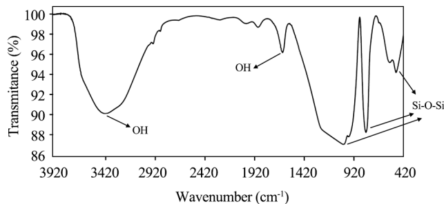
شکل ۳- طیف FTIR نکه‌دارنده سیلیکایی.
