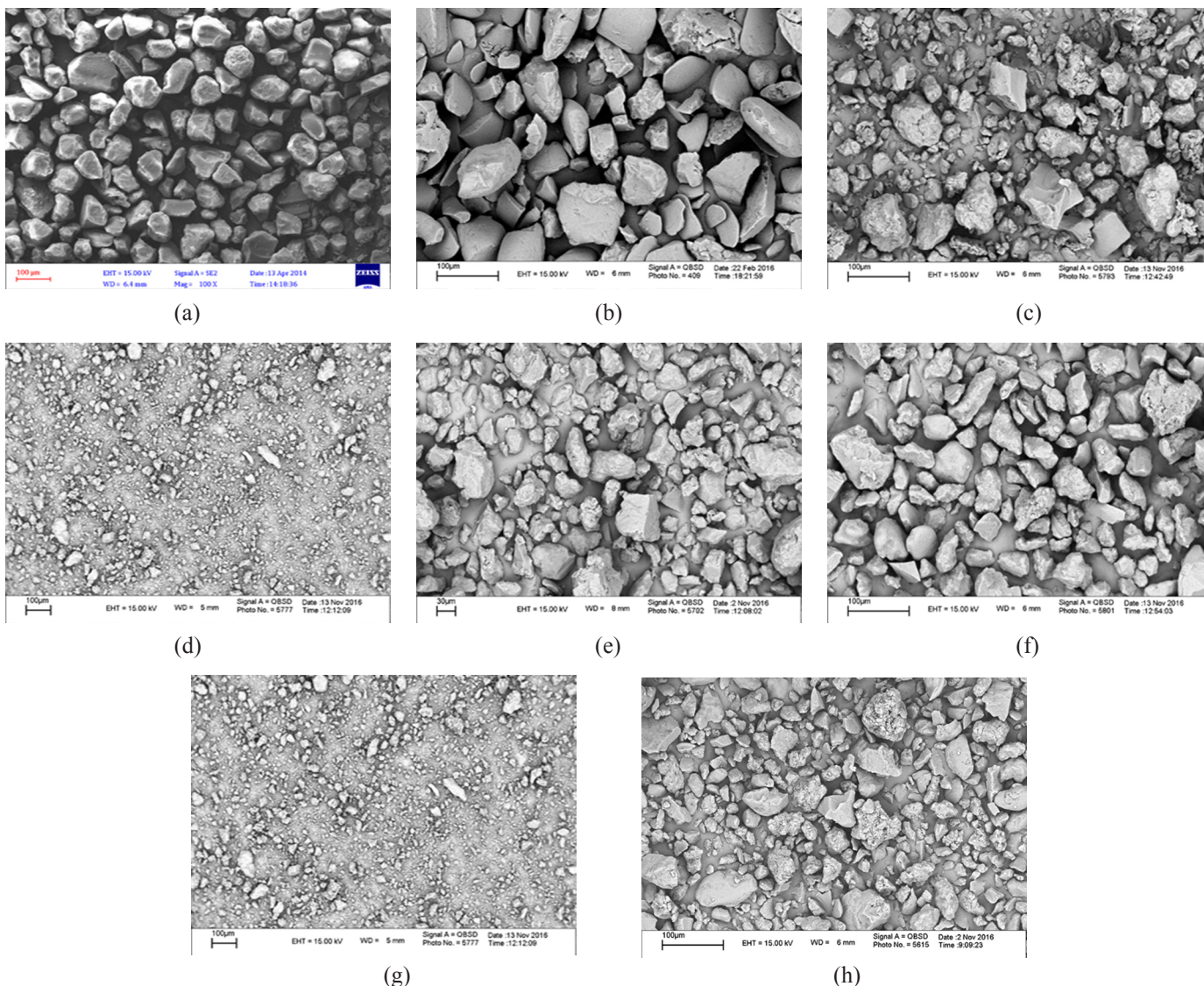
شکل ۴- عکس‌های SEM نگاه‌دارنده سیلیکایی سنتز شده با حلال‌های مختلف و کاتالیزگر آریاسول (C230) (با وضوح 100 \mu\text{m} ).
