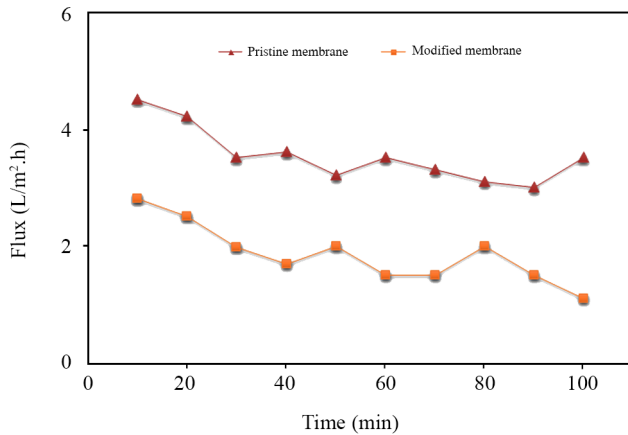
شکل ۸- شار محلول دارای فلزات سنگین برای غشای اولیه و نمونه غشای بهینه در شرایط محیطی و فشار ۵ bar.
