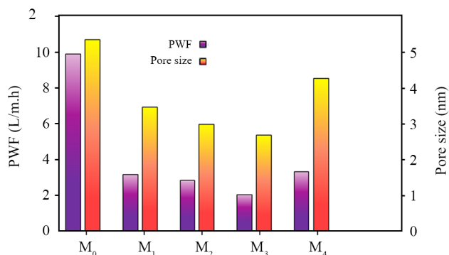
شکل ۵- اثر ایجاد لایه سطحی پلی (متیل متاکریلات) دارای مقادیر متفاوت از نانوصفحه‌های اکسید گرافن بر شار آب خالص (در فشار ۵ bar) و شعاع متوسط منفذها.
