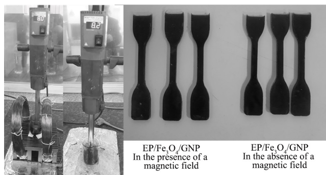
شکل ۳- نمایی از (a) میدان مغناطیسی و مخلوط‌کن با سرعت برش زیاد، (b) مخلوط‌کن با سرعت برش زیاد در کاربرد روش پراکنش نانوذرات و (c) نمونه‌های رزین تقویت‌شده.
