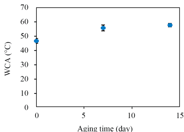
شکل ۷- اثر زمان نگهداری در ترشوندگی زیرلایه‌های پیوندخورده با PHEMA در زمان پلیمر شدن ۶ h و زمان پیش‌عمل‌آوری ۱۵ min. Fig. 7. Effect of storage time on the wettability of PHEMA-grafted substrates with a polymerization time of 6 h and a pretreatment time of 15 min.
