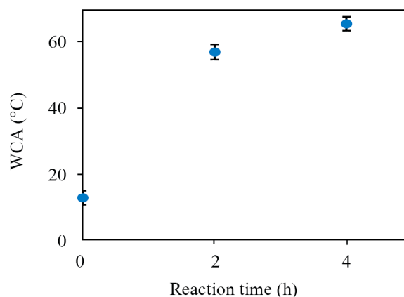
شکل ۳- اثر زمان غوطه‌وری زیرآیند پلی استیرنی عمل آوری شده با UVO به مدت ۱۵ min بر WCA سطح لایه‌نشانی شده با آغازگر.
