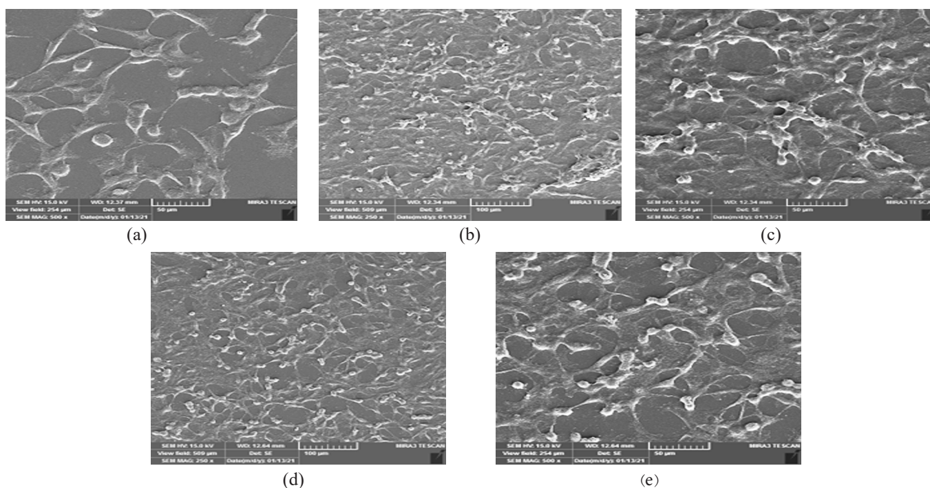
شکل ۸- تصاویر SEM مربوط به رفتار یاخته‌ای NIH3T3 روی سطوح مختلف: سطح PS عمل‌آوری‌نشده (a) و PS پیوندخورده با PHEMA به روش ATRP آغاز شده از سطح با زمان پلیمر شدن ۲ h (b و c، با دو بزرگنمایی مختلف) و زمان پلیمر شدن ۶ h (d و e، با دو بزرگنمایی مختلف). Fig. 8. SEM images showing NIH3T3 cell behavior on different PS surfaces: untreated PS surfaces (a) and PHEMA-grafted PS surfaces by surface-initiated ATRP with polymerization time of 2 h (b and c with different magnifications) and polymerization time of 6 h (d and e with different magnifications).
