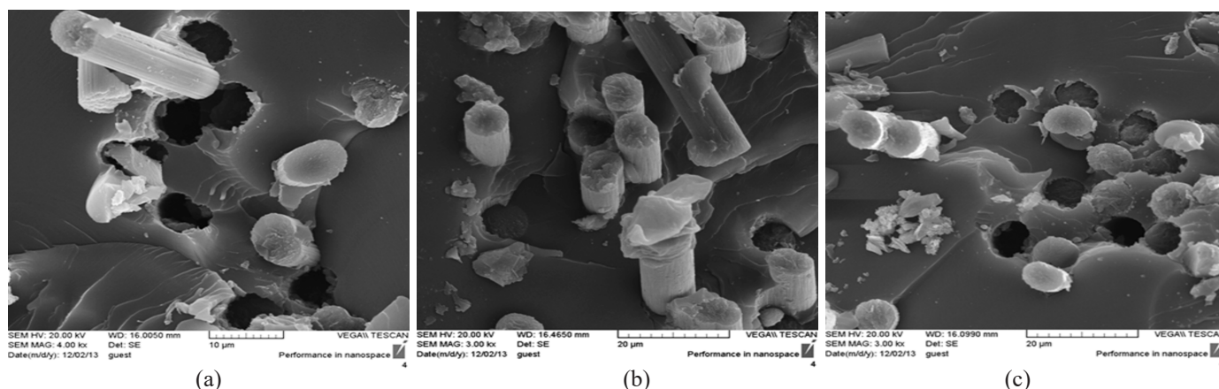
شکل ۶- تصاویر SEM از سطح شکست مواد کامپوزیتی تقویت شده با (a) الیاف کربن اکسید نشده و الیاف کربن اکسید شده به وسیله الکترولیت های \text{HNO}_3 (b) و \text{NaOH} (c).
