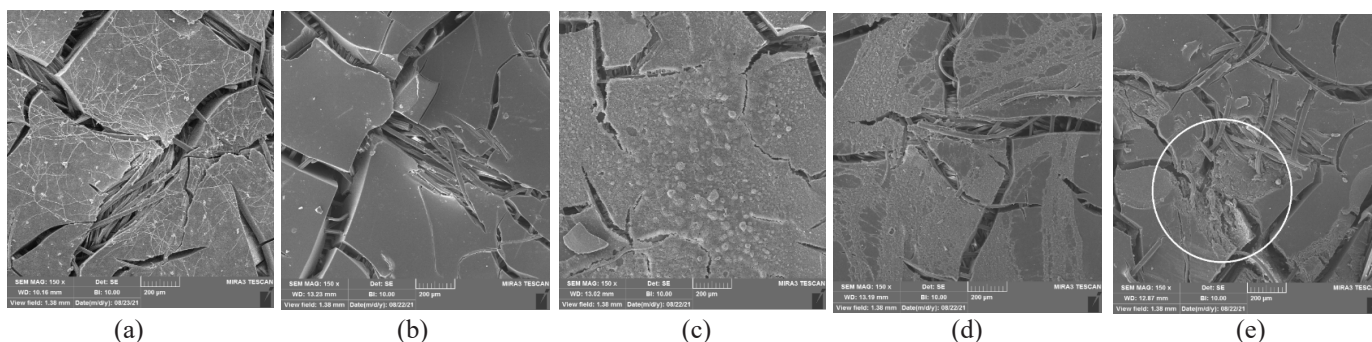
شکل ۲- تصاویر SEM از سطح غشاها: (a) غشای پایه، (b) غشای اصلاح‌شده با لایه لاستیکی و غشای اصلاح‌شده با لایه لاستیکی دارای نانوذرات گرافیت (c) ۰/۱٪ وزنی، (d) ۱٪ وزنی، (e) ۱۰٪ وزنی.
