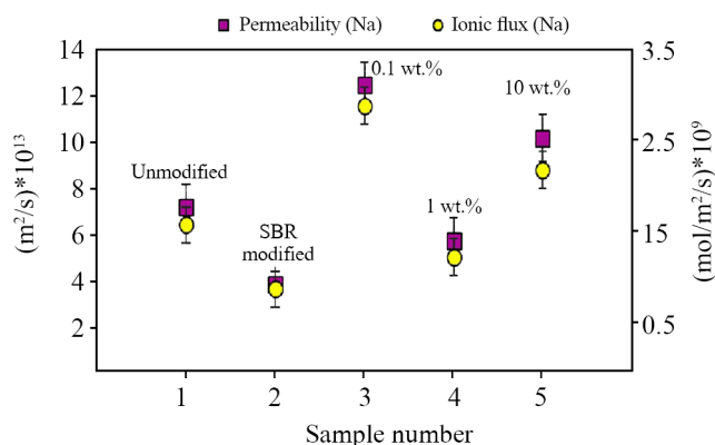
شکل ۹- تراوایی و شار یونی غشاهای ساخته شده. Fig. 9. Permeability and ionic flux for the prepared membranes.
