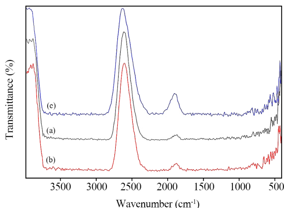
شکل ۶- نتایج FTIR برای غشاهای تهیه شده: (a) غشای پایه، (b) غشای اصلاح شده با لایه لاستیکی و (c) غشای اصلاح شده با لایه لاستیکی دارای نانوذرات گرافیت.
