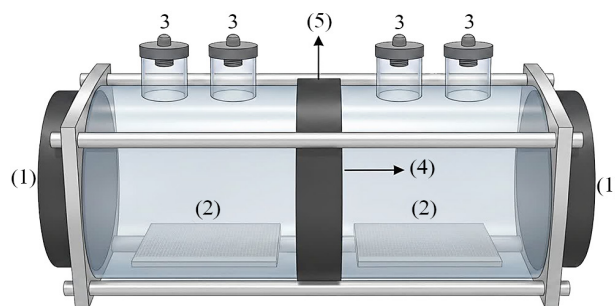
شکل ۱- تصویر دستگاه غشایی الکترو دیالیز.
