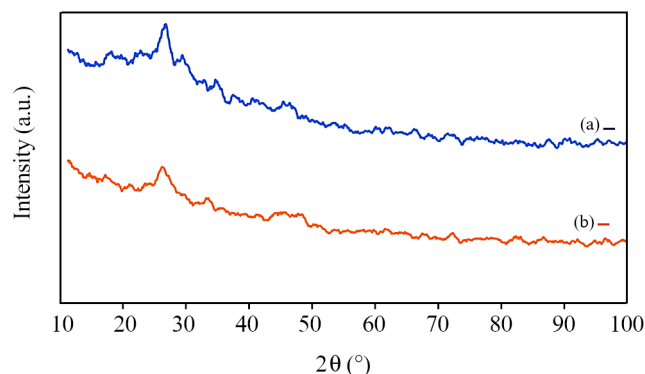
شکل ۵- آزمون پراش پرتو X از غشاهای تهیه شده: (a) غشای پایه و (b) غشای اصلاح شده با لایه لاستیکی دارای نانوذرات گرافیت.
