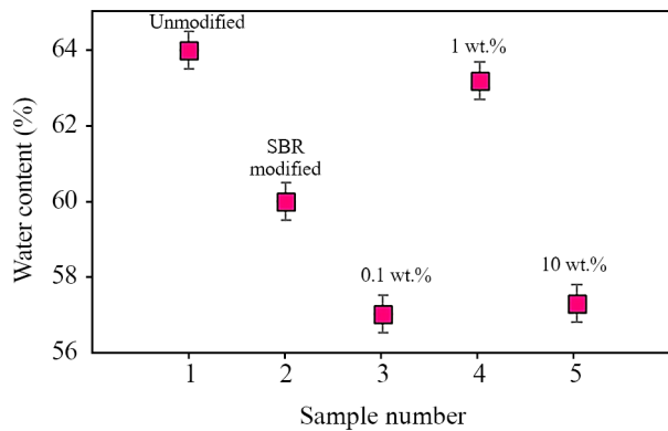
شکل ۸- اثر اصلاح سطحی بر مقدار محتوای آب غشاهای تهیه شده. Fig. 8. The effect of surface modification on the water content of the prepared membranes.
