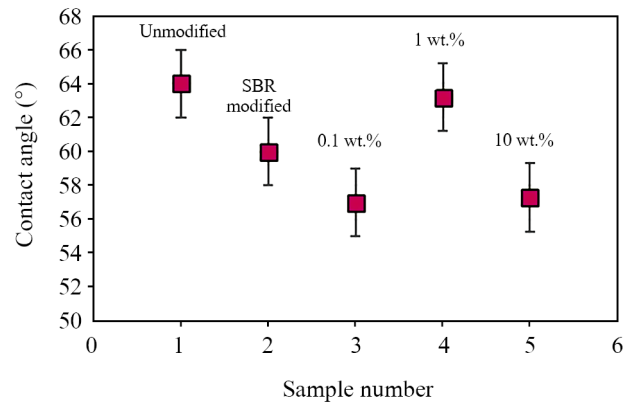
شکل ۷- نتایج اندازه‌گیری زاویه تماس برای غشاهای تهیه شده. Fig. 7. The contact angel measurement for the prepared membranes.
