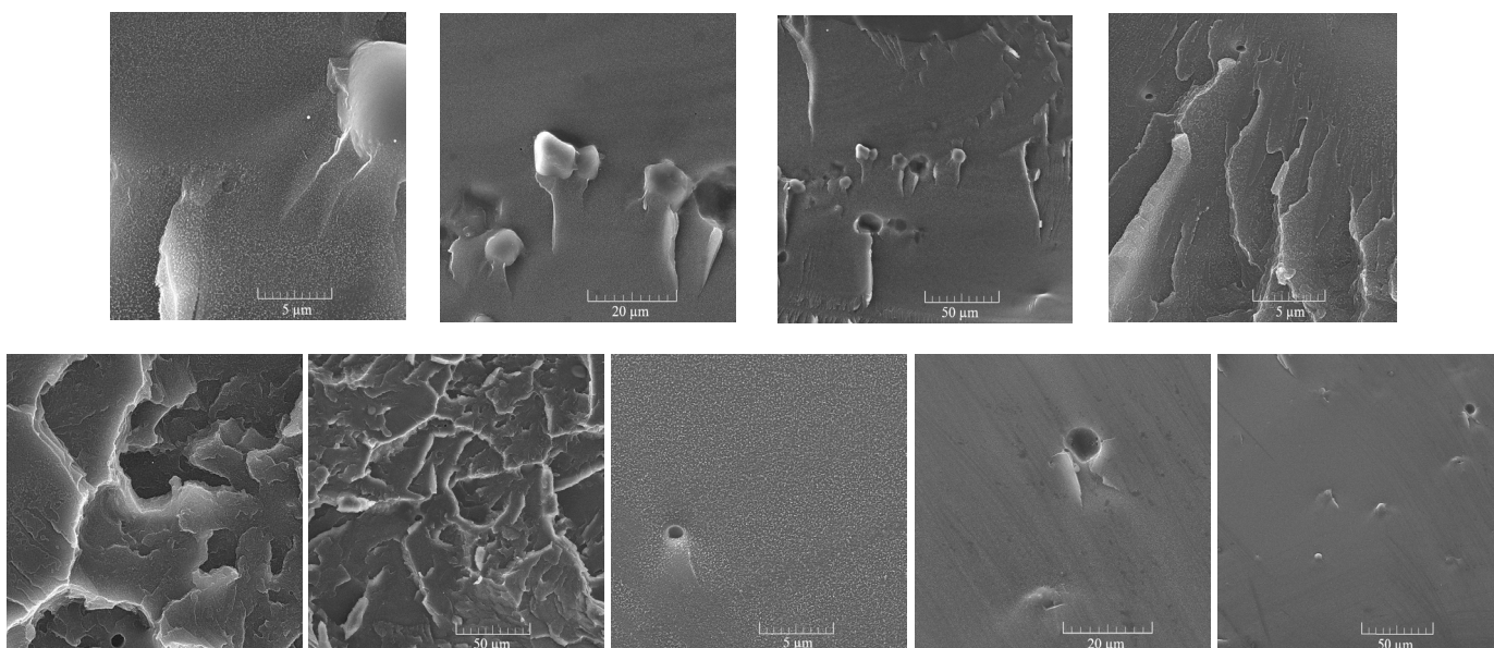
شکل ۵- تصاویر FE-SEM نمونه‌های PS، PSPa3 و PSPa30 پس از تخریب.
