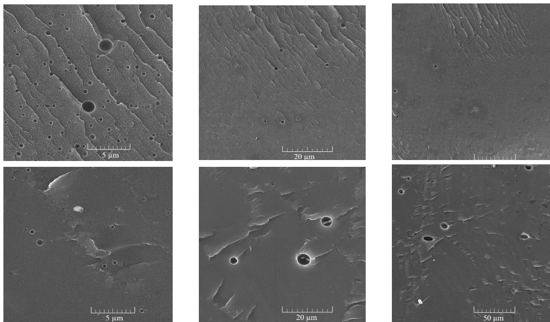
شکل ۶- تصاویر FE-SEM نمونه های PSSSt3, PSSSt3O پس از تخریب.
