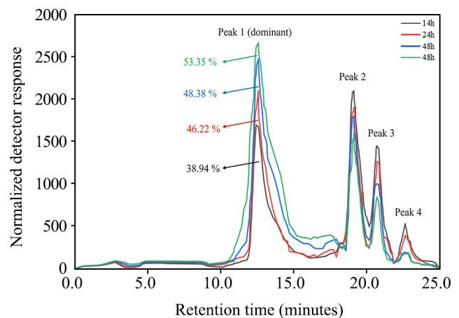
شکل ۴- طیف های GPC \gamma\text{-PGA} تولید شده در زمان های مختلف تخمیر. Fig. 4. GPC spectra of produced \gamma\text{-PGA} at different fermentation times.
