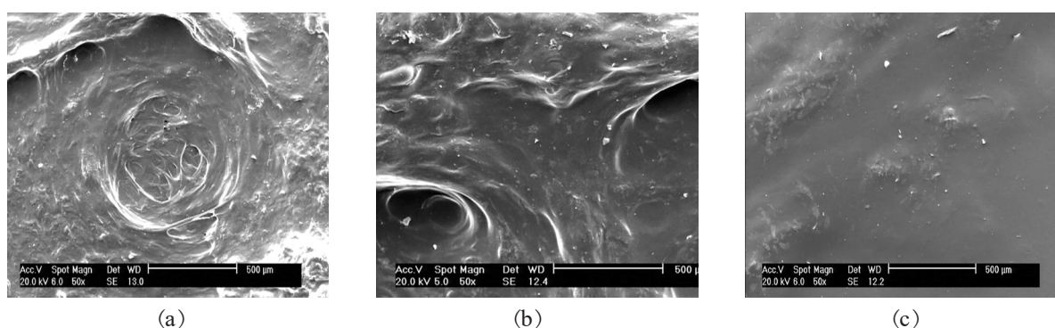
شکل ۳- تصاویر SEM هیدروژل‌های دوجزئی کتیرا/کتوسان (Tg/Cs) با نسبت‌های مختلف: (a) ۳۰/۷۰، (b) ۵۰/۵۰ و (c) ۷۰/۳۰؛ شبکه‌ای شده با ۱/۵٪ \text{CaCl}_2 ؛ بزرگ‌نمایی ۵۰x.
