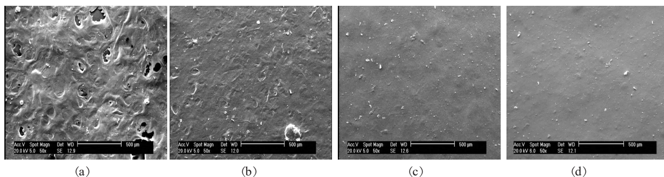
شکل ۲- تصاویر SEM هیدروژل‌های دوجزئی کتیرا/آلژینات (Tg/Alg) با نسبت‌های مختلف: (a) ۰/۱۰۰، (b) ۳۰/۷۰، (c) ۵۰/۵۰ و (d) ۷۰/۳۰؛ شبکه‌ای شده با ۱/۵٪ \text{CaCl}_2 ؛ بزرگ‌نمایی ۵۰x.
