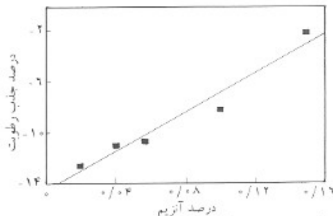
شکل ۷- اثر غلظت آزریم بر میزان جذب رطوبت.
