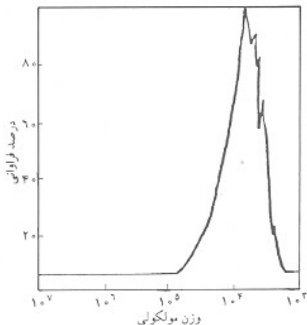
شکل ۱- منحنی توزیع وزن مولکولی موم HDPE
