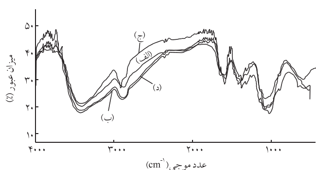
شکل ۲ - مقایسه طیفهای FTIR نمونه های کیتوسان: (الف) استاندارد آلد ریچ، (ب) پوسته خرچنگ، (ج) پوسته سیست آرتمیا اورمیا و (د) پوسته میگو.
