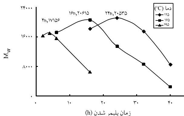
شکل ۲- اثر دما و زمان واکنش بر متوسط وزنی وزن مولکولی پلی (L-لاکتید).
