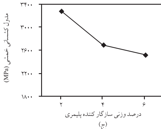
شکل ۱- آثار اصلی عوامل مختلف بر پاسخ مدول کشسانی خمشی: (الف) اثر درصد وزنی PP/HDPE، (ب) اثر درصد وزنی MAPP، (ج) اثر درصد وزنی سازگار کننده پلیمری و (د) اثر نوع سازگار کننده پلیمری.
