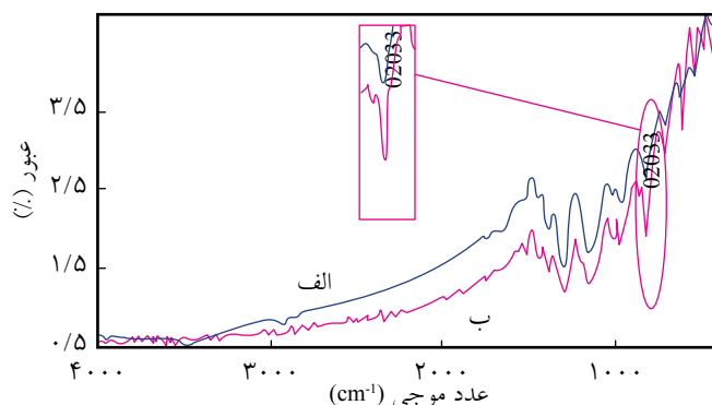
شکل ۱- طیف FTIR: (الف) پودر پلی (۳- متیل تیوفن) و (ب) ذرات پلیمری جدا شده از سطح پلی استر.
