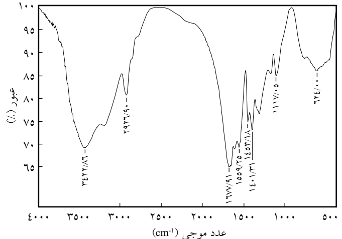
شکل ۱- طیف زیرقرمز پلی‌آکریل‌آمید آنیونی تهیه شده با ۳۰ درصد آب‌کافت.
