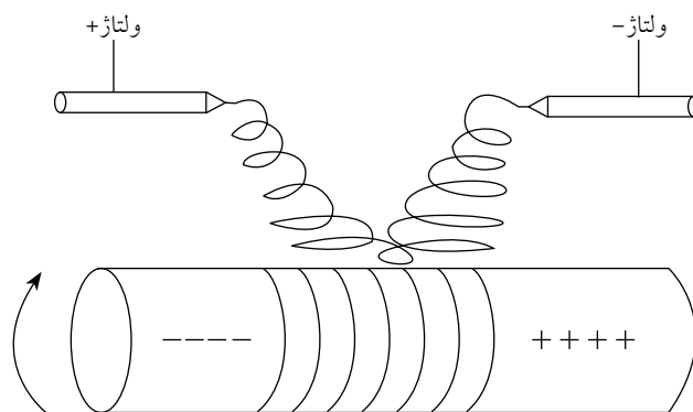
شکل ۱- طرح کلی نحوه تولید نانوالیاف موازی با استفاده از دو سوزن الکتروریسی و یک غلتک جمع‌کننده.
