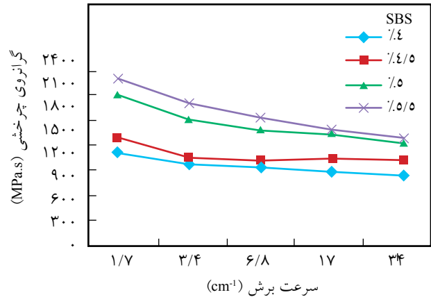
شکل ۲- نمودار گرانروی چرخشی بر حسب سرعت برش برای درصدهای مختلف SBS با ۲۵ درصد VB.
