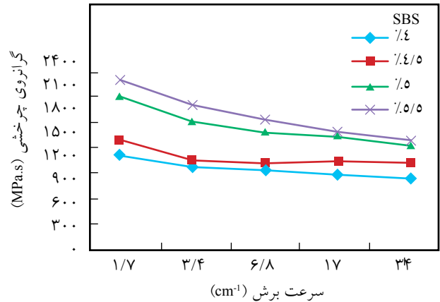
شکل ۲- نمودار گرانروی چرخشی بر حسب سرعت برش برای درصدهای مختلف SBS با ۲۵ درصد VB.
