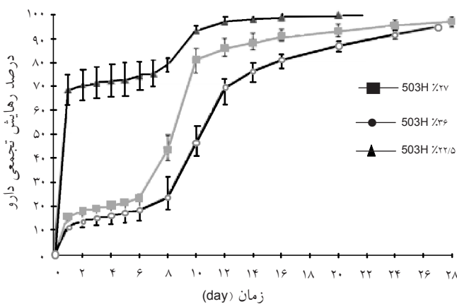
شکل ۷- منحنی‌های رهایش دارو از سامانه‌های با ترکیب داکسی سائیکلین هیكلیت: PLGA:NMP و با نسبت‌های وزنی ۱۰:۵۴:۳۶، ۱۰:۶۳:۲۷ و ۱۰:۶۷:۲۲/۵.
