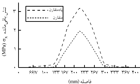
شکل ۸ - اثر زاویه الیاف در نمونه [۰/۳۰/۳۰/۳۰/۰] (با مجوز ناشر مرجع [۳۴]).
