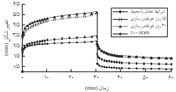
شکل ۴- اثر زمان غوطه‌ورسازی بر خزش کامپوزیت‌های چوب - پلیاستیک (مقدار ۶۰٪ آرد MDF).
