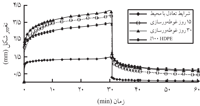
شکل ۶- اثر زمان غوطه‌ورسازی بر خزش کامپوزیت‌های چوب - پلیاستیک (مقدار ۸۰٪ آرد MDF).
