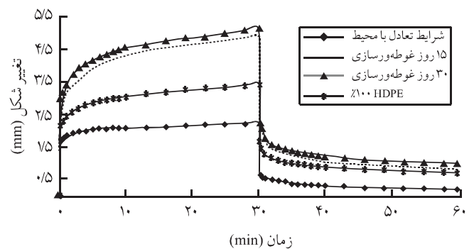
شکل ۵- اثر زمان غوطه‌ورسازی بر خزش کامپوزیت‌های چوب - پلیاستیک (مقدار ۷۰٪ آرد MDF).
