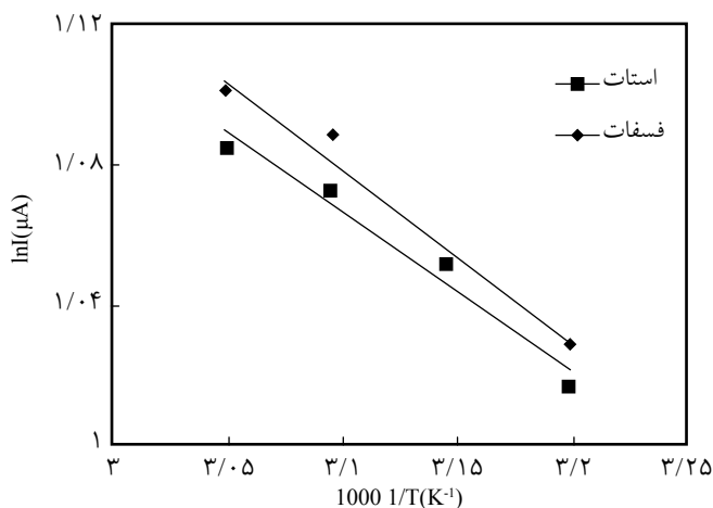
شکل ۱۲- نمودار \ln I بر حسب 1/T برای الکتروود اصلاح شده در محیط بافری فسفات و استات.
