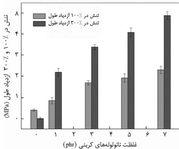
شکل ۶- مقایسه تشنش در ۱۰۰٪ و ۳۰۰٪ ازدیاد طول کامپوزیت‌های EPDM/MWCNT سازگار شده حاوی غلظت‌های مختلف نانولوله‌های کربنی.
