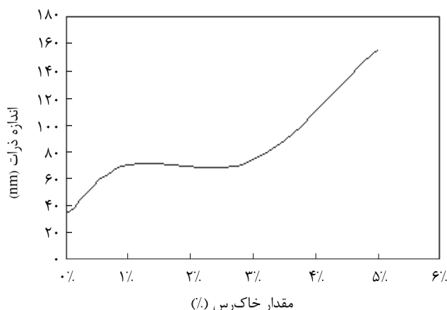
شکل ۱- تغییرات اندازه ذرات امولسیونی با مقدار نانوخاک‌رس.
