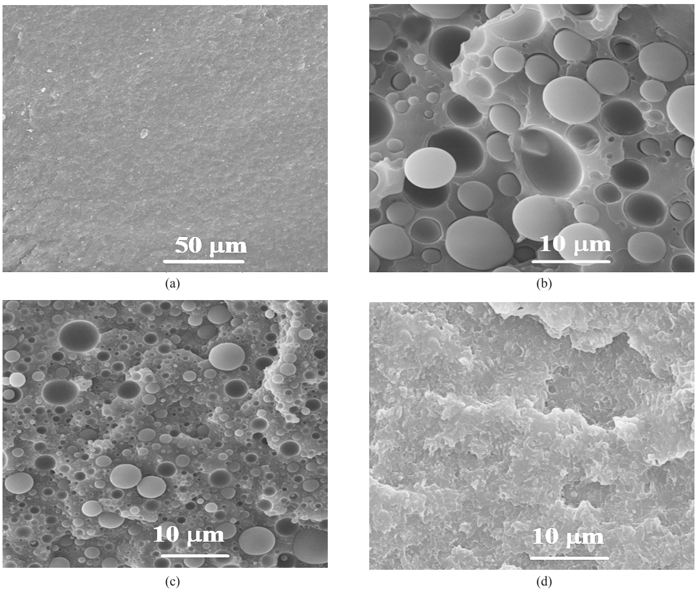
شکل ۳- عکس‌های SEM از سطح شکست سرمایشی نمونه‌ها: (a) خالص PLA، (b) PLA/EVA، (c) PLA/EVA/R5، و (d) PLA/EVA/R10. Fig. 3. SEM images of cryo-fractured surface of samples: (a) neat PLA, (b) PLA/EVA, (c) PLA/EVA/R5, and (d) PLA/EVA/R10.
