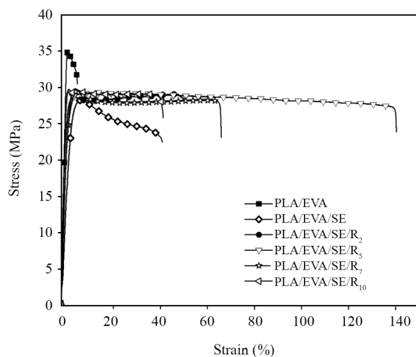
شکل ۸- منحنی‌های تنش-کرنش آمیخته سازگار شده PLA/EVA دارای مقادیر مختلف نانو سیلیکا.
