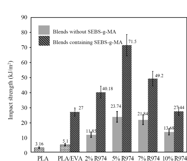
شکل ۹- استحکام ضربه‌ای آیزود شکاف‌دار در نمونه‌های مختلف. Fig. 9. Notched Izod impact strength of different samples.
