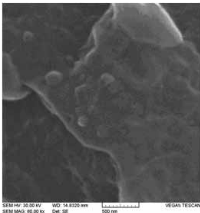
شکل ۲- تصویر میکروسکوپ الکترونی پوششی کامپوزیت PVDF-5%N6-3%Coisite 30B
