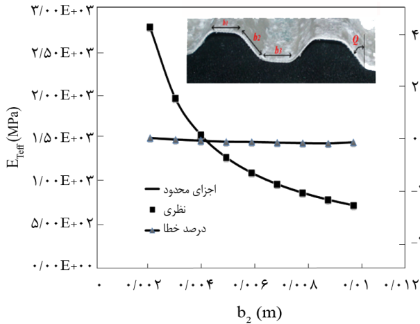
شکل ۱۳- مقایسه نتایج اجزای محدود و تحلیلی (سفتی کششی مؤثر در راستای عرضی بر حسب b_2 ).
