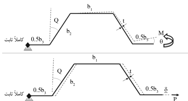
شکل ۴- اجزای دوزنقه‌ای زیر بار کششی و ممان خمشی.
