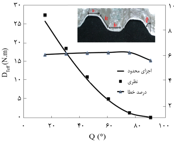
شکل ۱۵- مقایسه نتایج اجزای محدود و تحلیلی (سفتی خمشی مؤثر در راستای عرضی بر حسب Q ).
