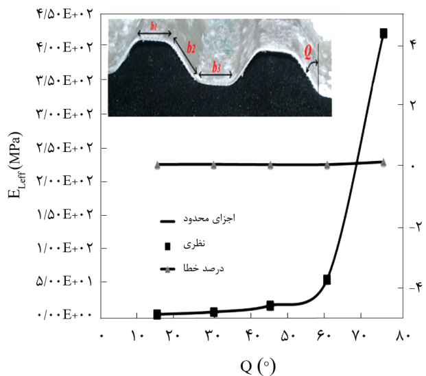
شکل ۱۲- مقایسه نتایج اجزای محدود و تحلیلی (سفتی کششی مؤثر در راستای طولی بر حسب Q ).
