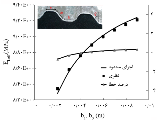
شکل ۱۱- مقایسه نتایج اجزای محدود و تحلیلی (سفتی کششی مؤثر در راستای طولی بر حسب b_1 و b_3 ).
