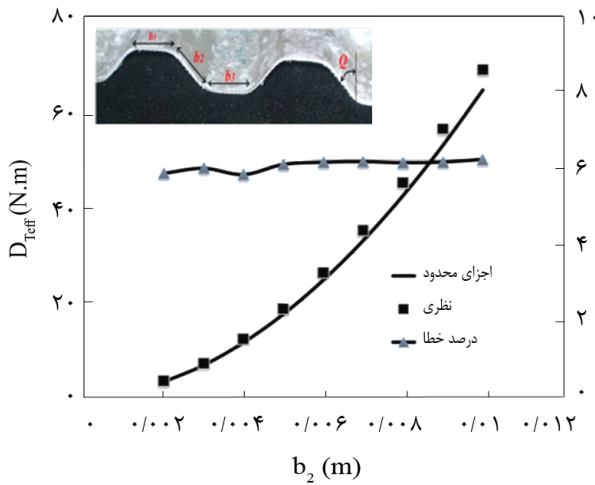
شکل ۱۴- مقایسه نتایج اجزای محدود و تحلیلی (سفتی خمشی مؤثر در راستای عرضی بر حسب b_2 ).
