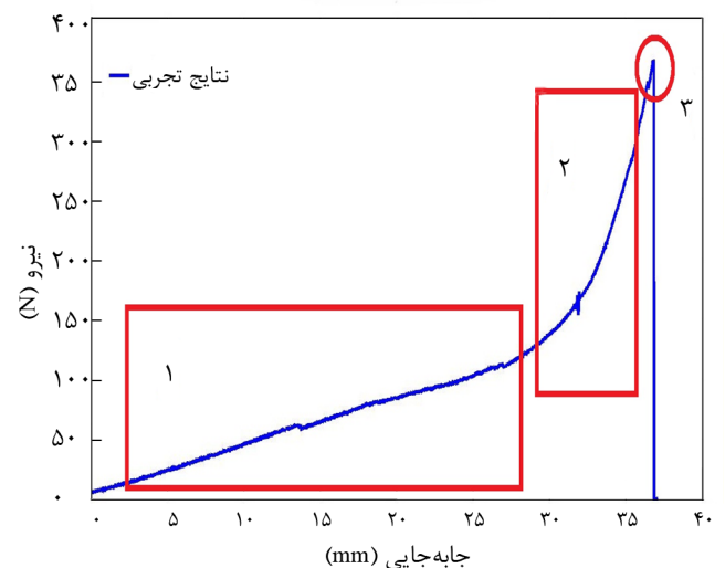
شکل ۲۱- آزمون کشش برای نمونه دوزنقه‌ای ( b_1=b_3=5 mm, b_2=8 mm و Q=45^\circ ).
