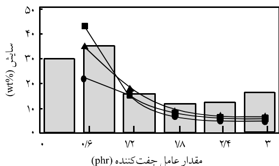
شکل ۵ - اثر فرمولبندی، نوع و مقدار عوامل جفت کننده بر مقاومت سایشی آمیزه ها: (□) کنترل، (●) سیلان، (■) HVA-2 و (▲) رنوفیت.
