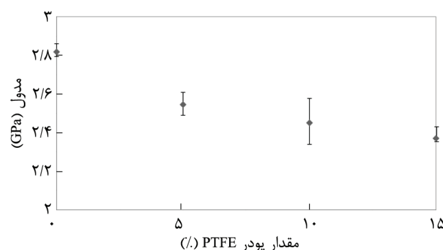
شکل ۴- اثر مقدار پودر PTFE پرتودهی شده بر مدول کامپوزیت‌ها.
