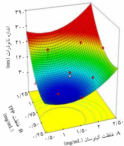
شکل ۱- نمودار سه‌بعدی مدل مربوط به اندازه ذرات.
