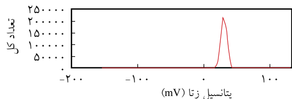
شکل ۵- نمودار توزیع بار سطحی نانوذرات در شرایط پهنه.
