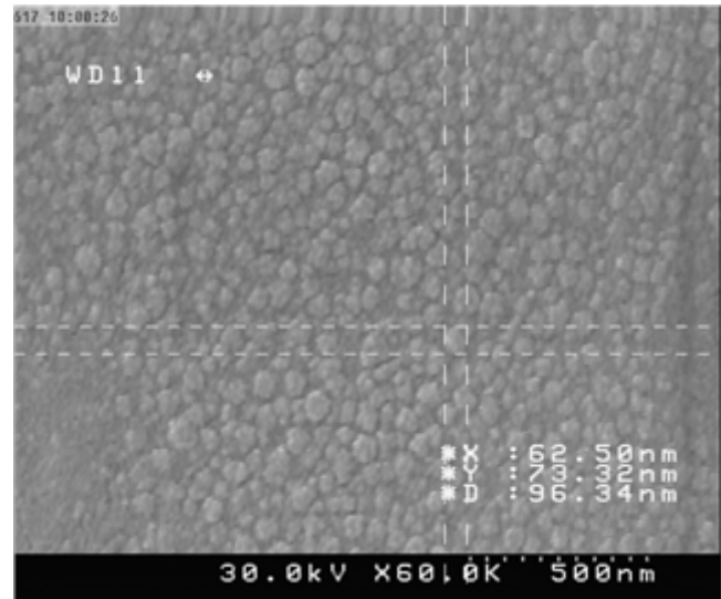
شکل ۴- تصویر FESEM مربوط به نانوذرات در شرایط پهنه متغیرها.
