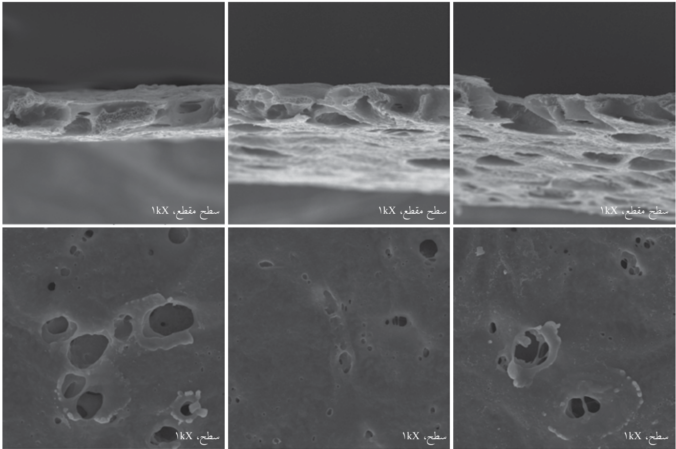
شکل ۶- تصاویر سطح مقطع و سطح غشاهای تشکیل شده از ۱۲٪ PES، با دمای 20 \pm 45^\circ\text{C} و رطوبت نسبی ۷۰٪ در محیط تأخیر، در زمان‌های نامند: (الف) ۵ min، (ب) ۱۰ min و (ج) ۲۰ min.
