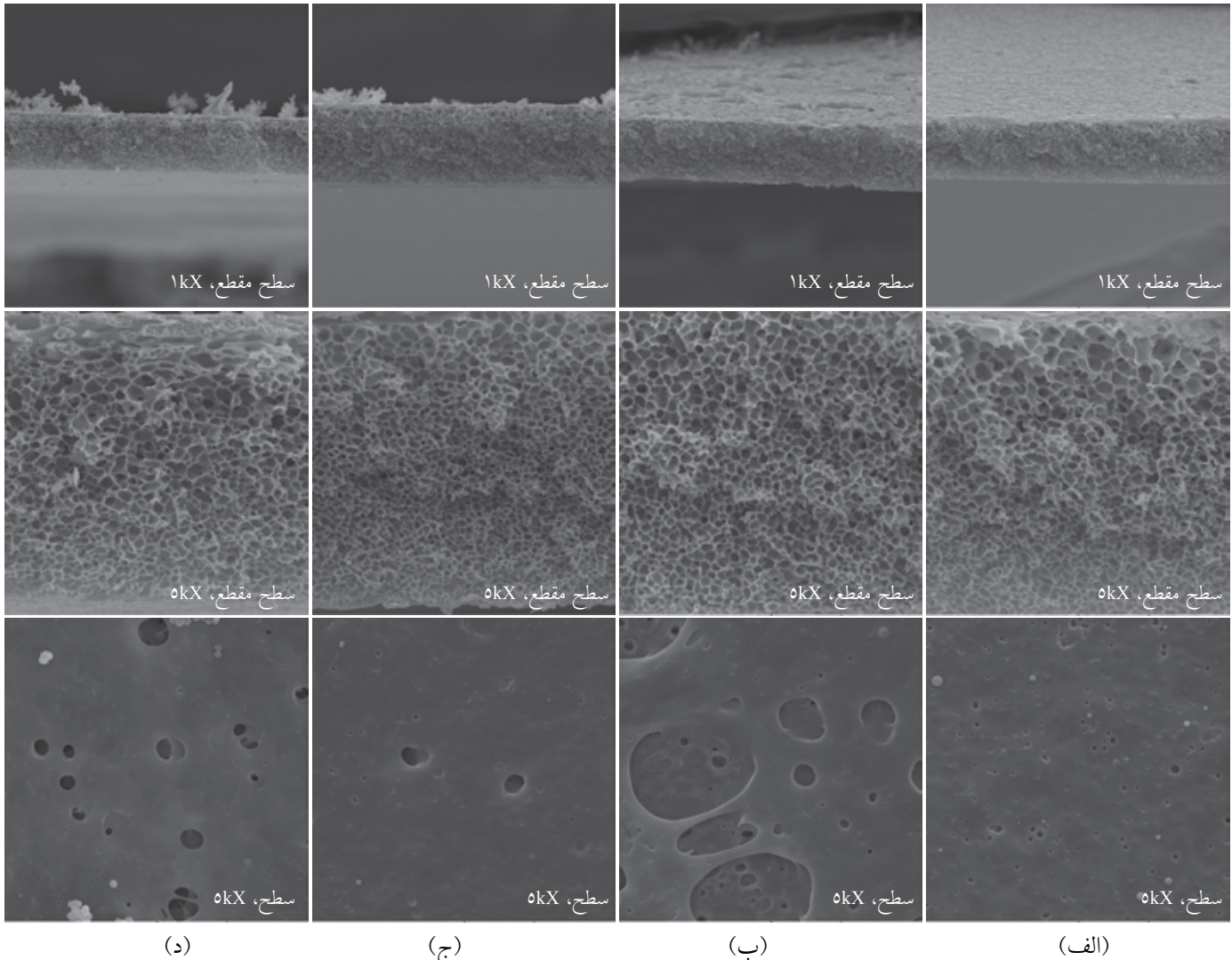
شکل ۸- تصاویر سطح مقطع در دو بزرگ نمایی و سطح غشاهای تشکیل شده از ۱۵٪ PES، با دمای 20 \pm 45^\circ\text{C} و رطوبت نسبی ۷۰٪ در محیط تأخیر، با غلظت‌های: (الف) ۵٪، (ب) ۷/۵٪، (ج) ۱۰٪ و (د) ۱۲/۵٪ از افزودنی PVP K17.
