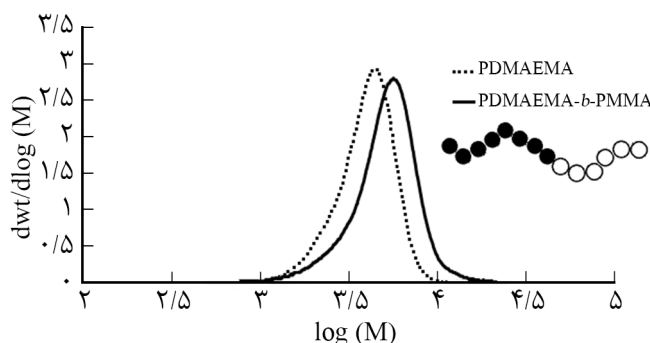
شکل ۳- نمودار GPC برای PDMAEMA و PDMAEMA- b -PMMA تهیه شده در دو مرحله پلیمر شدن RAFT.
