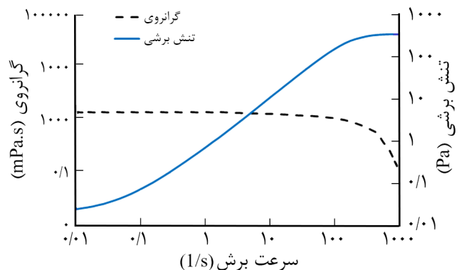
شکل ۹- رفتار رئولوژی محلول آبی SDS-DMAPA با تغییرات گرانی بر حسب سرعت برش و تنش برشی.
