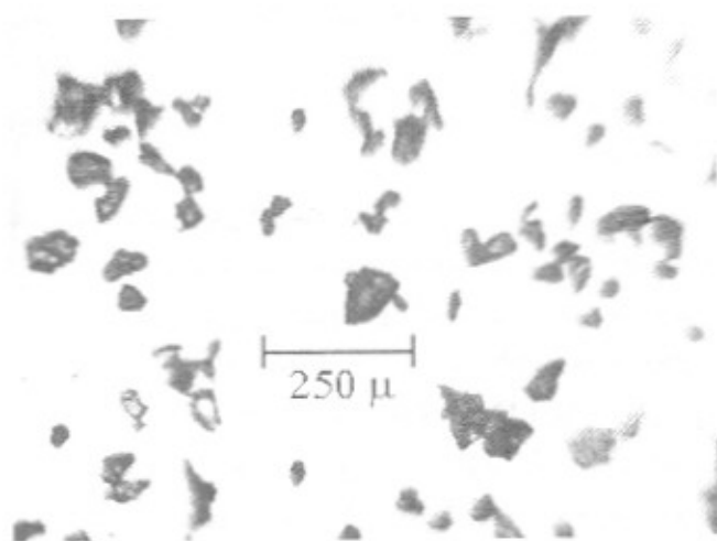
شکل ۳- ذرات هیدروژل آکریلیک اسید پس از عبور از الک با اندازه روزنه ۱۲۰ μ.
