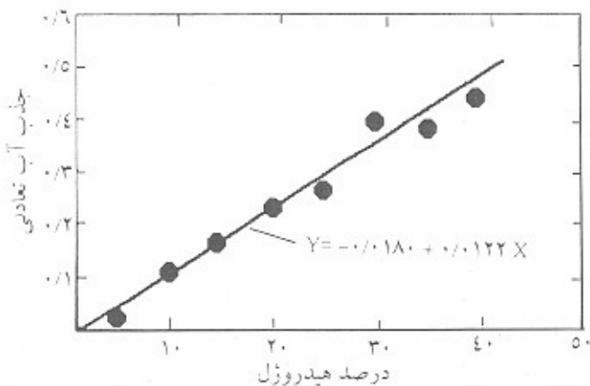
شکل ۶- رابطه میان درصد هیدروژل با میزان جذب آب تعادلی (پلی آکرلیک اسید با میزان عامل شبکه ای کننده ثابت و مطابق فرمولبندی جدول ۲ تهیه شد).
