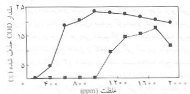
شکل ۲- میزان حذف COD در pH ثابت نسبت به غلظت مواد منعقد کننده: آهن (III) سولفات (●) و کلسیم هیدروکسید (■).
