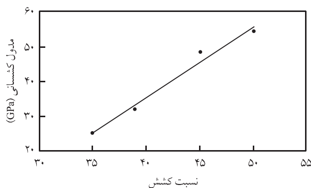
شکل ۷ تغییرات مدول کشسانی با نسبت کشش.
