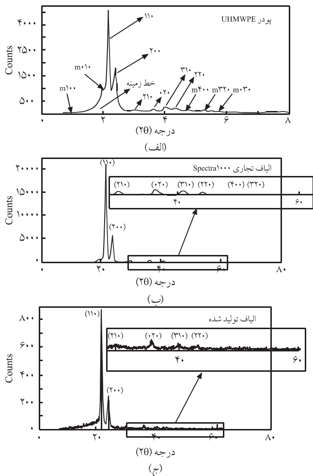
شکل ۵ نمودار پراش پرتو X: (الف) پودر UHMWPE، (ب) الیاف Spectra 1000 و (ج) الیاف تولید شده.
