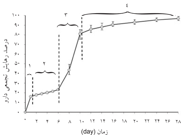
شکل ۶- منحنی رهایش دارو از سامانه با ترکیب داکسی سایکلین هیکلیت: PLGA: NMP با نسبت وزنی ۱۰:۶۳:۲۷.
