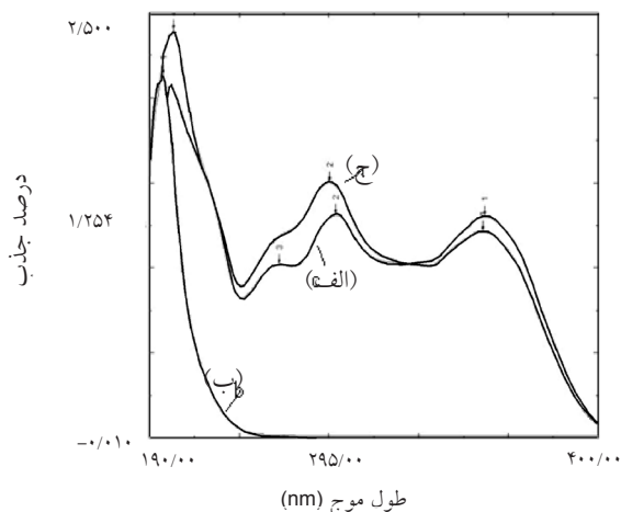
شکل ۴- طیف های UV: (الف) محلول حاوی ۵۰ ppm داکسی سایکلین هیکلیت، (ب) محلول حاوی ۵۰ ppm از SMB و (ج) محلول حاوی ۴۰ ppm داکسی سایکلین هیکلیت و ۵۰ ppm از SMB.
