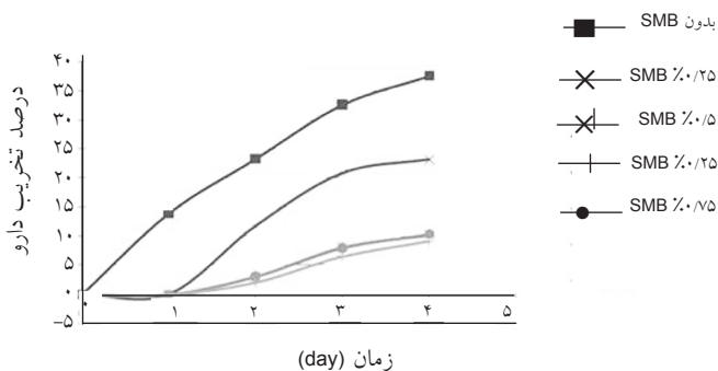
شکل ۵- اثر غلظت های مختلف افزودنی سدیم متابی سولفیت در مقدار تخریب داروی داکسی سایکلین هیکلیت در PBS و دمای ۳۷ °C
