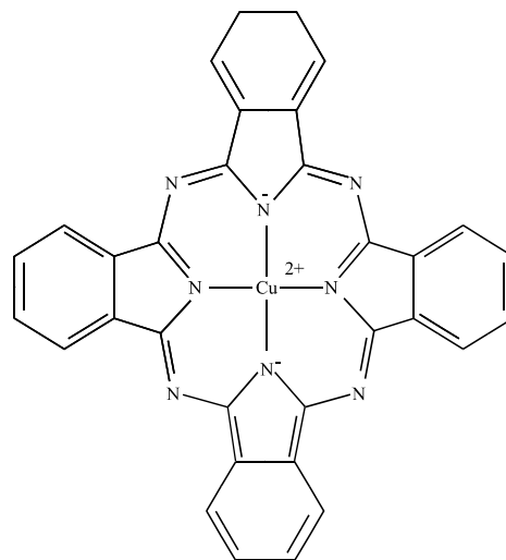
شکل ۱- ساختار شیمیایی رنگدانه به کار گرفته شده.
