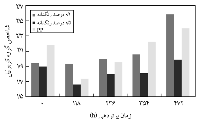
شکل ۱۲- تغییرات شاخص گروه کربونیل در نمونه‌های فیلم پلی‌پروپیلن محتوی رنگدانه در زمان‌های مختلف پرتودهی.
