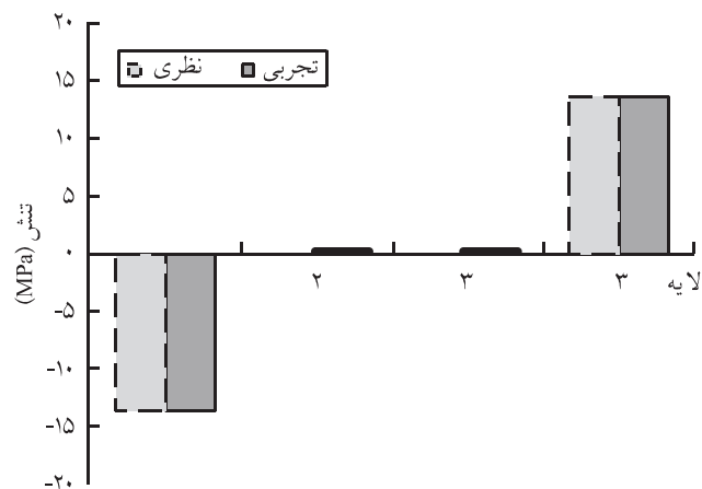
شکل ۳ - مقایسه نتایج تحلیلی و تجربی مولفه تنش \sigma_x در هر لایه از چندلایه‌های [0/\pm 45/90] .
