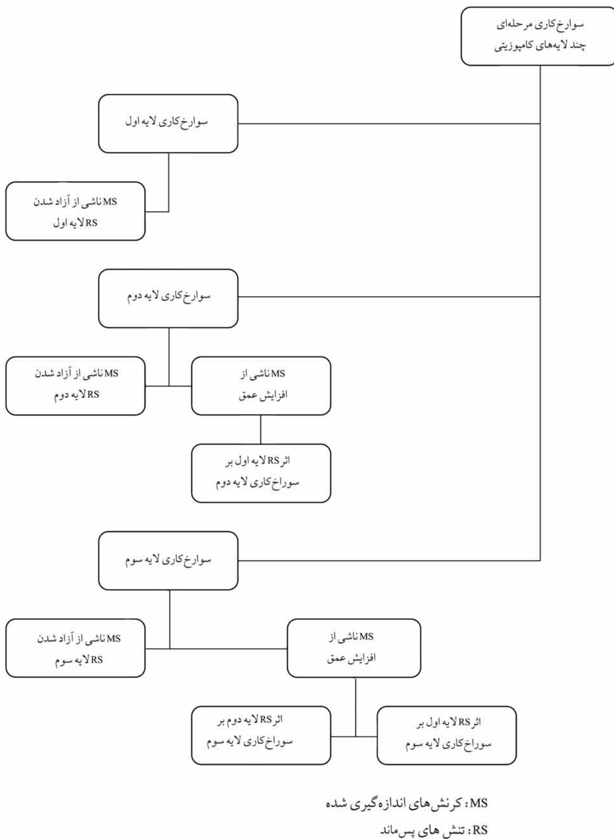
شکل ۲- ارتباط میان کرنش‌های اندازه‌گیری شده و تنش‌های پس ماند در روش سواری کاری مرحله‌ای.
